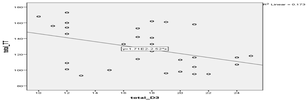
نمودار ۷ خط رگرسیون رابطه تعهد زناشویی و دلبستگی نایمن اجتنابی
